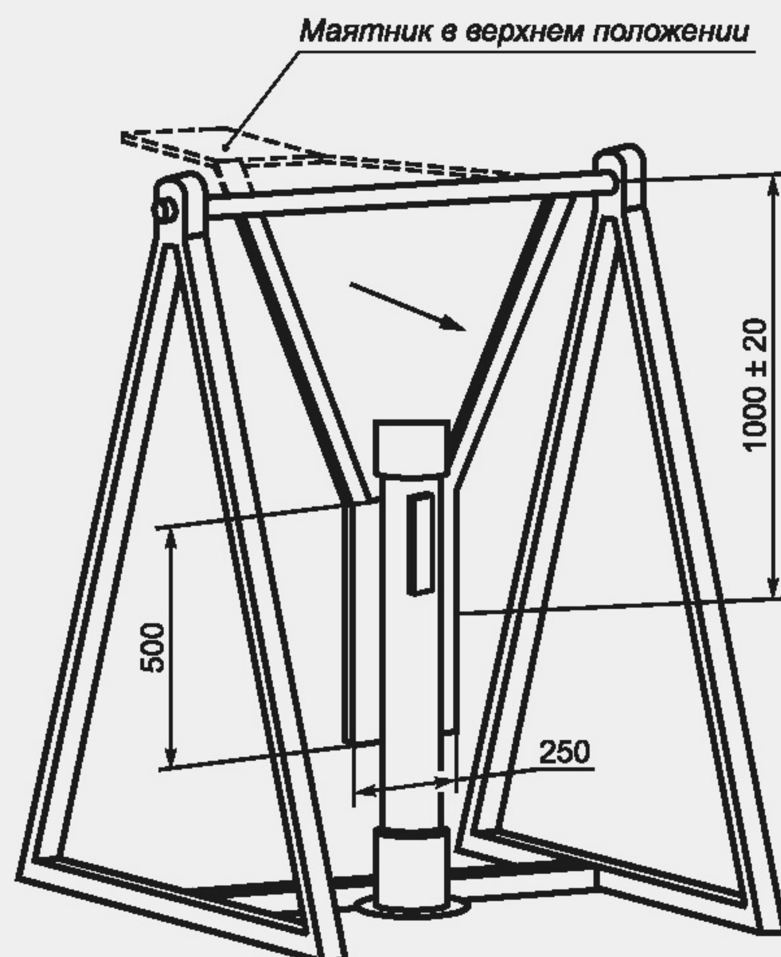
Рисунок 11 — Схема установки маятникового типа
